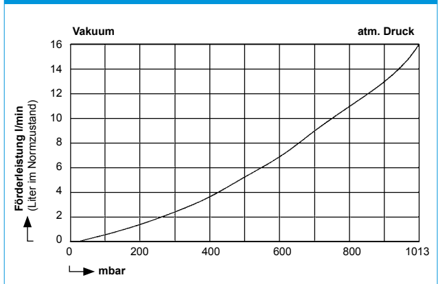
FÖRDERLEISTUNGSKURVE
